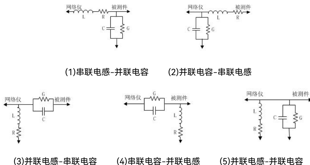
图 7.35 嵌入匹配电路的 5 种电路参数模型
