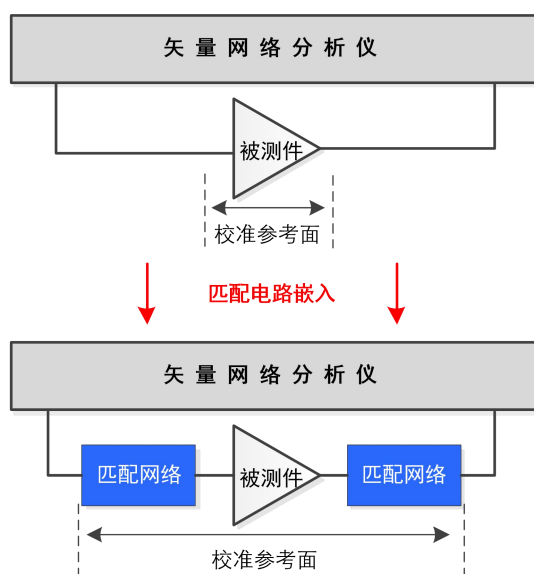
图 7.32 匹配电路嵌入示意图
