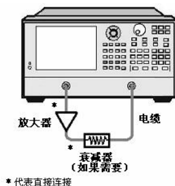
图 8.19 AM-PM 变换测量连接
