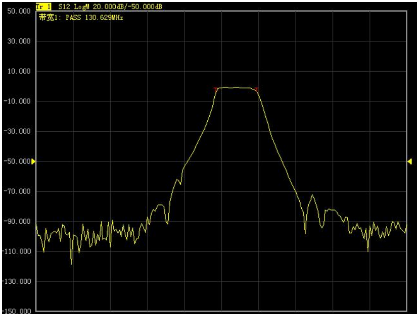
图 3.60 带宽测试显示结果
