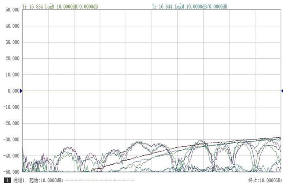
附图 4.28 平衡参数提取及四端口去嵌的结果
