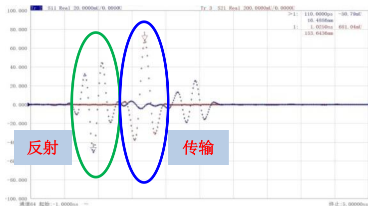
附图 4.7 反射参数和传输参数的时域变换
