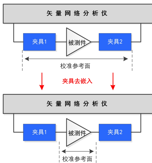
图 7.36 夹具去嵌入示例图
