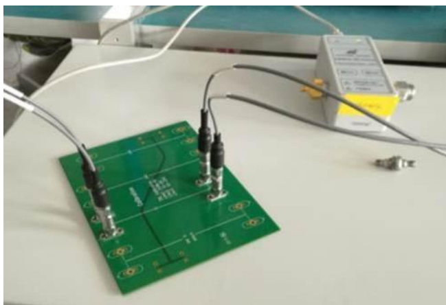
附图 4.25 差分夹具
