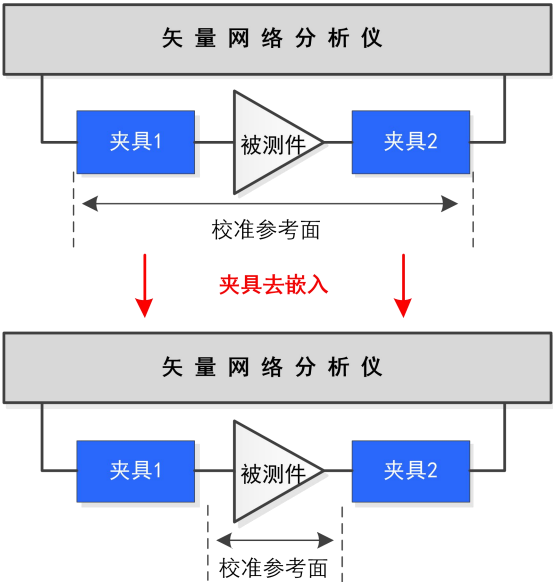
附图 4.9 夹具去嵌入示例图
