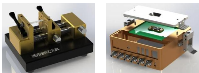
附图 4.4 通用微带测试夹具和芯片测试夹具
