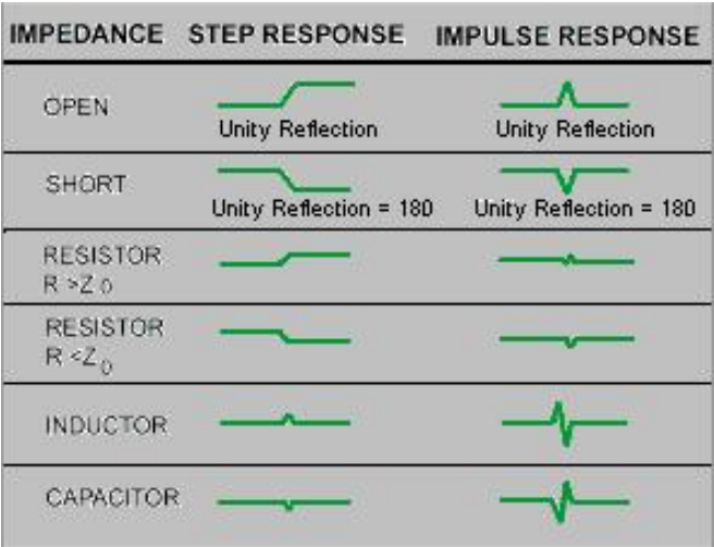
附图 2.18 不连续电路的低通时域响应波形
