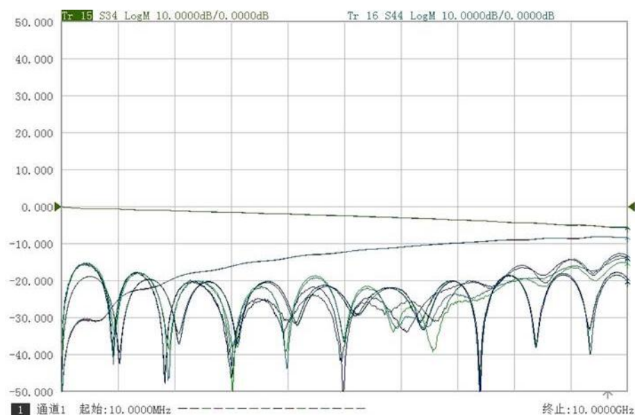
附图 4.26 差分夹具直通的原始参数
