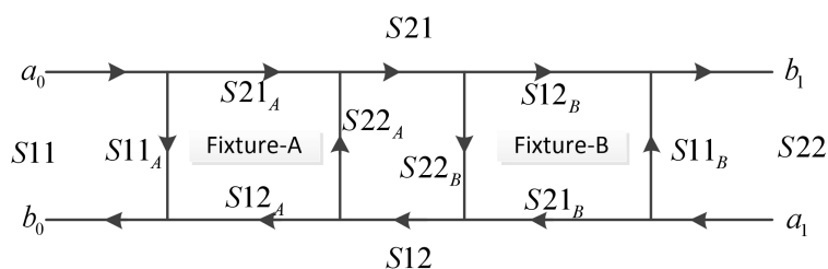
附图 4.6 直通标准的信号流图
