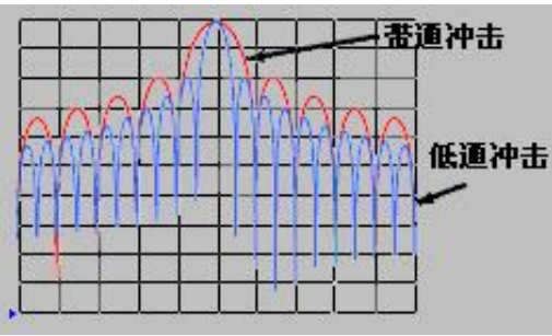
附图 4.14 变换模式对分辨率的影响
