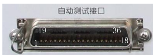
图3.35 自动测试接口连接器
