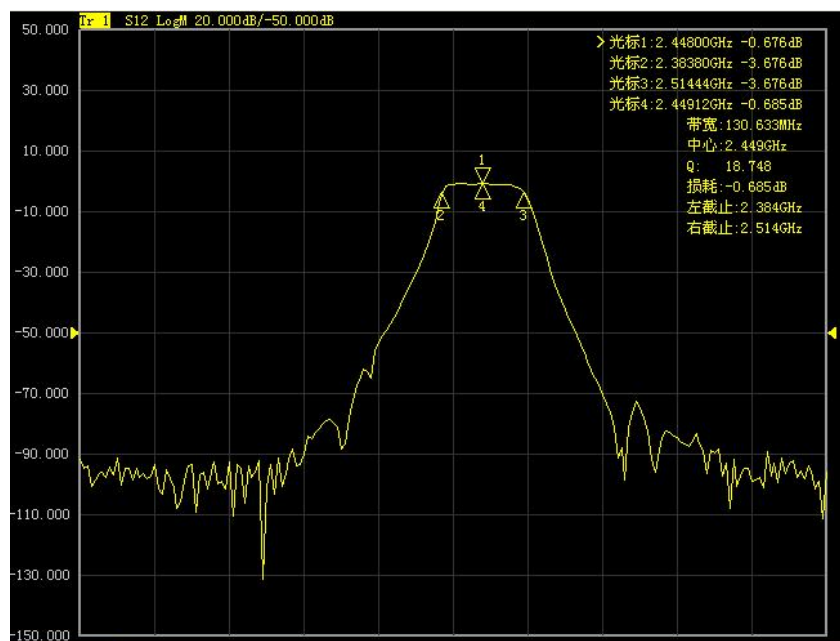
图 3.46 带宽搜索
