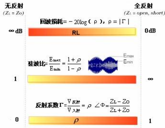
图8.6 各种反射表达之间的关系
