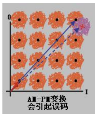
图 8.18 AM-PM 变换引起误码
