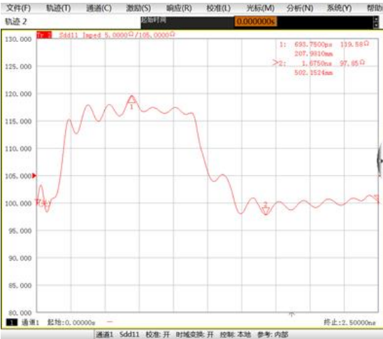
附图 2.31 时域反射（TDR）阻抗显示
