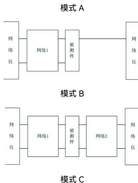
图 7.40 夹具嵌入/去嵌入的 3 种模式
