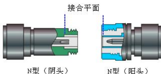
图 3.8 校准平面
