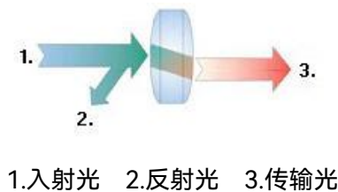
图 8.1 光的反射和传输
