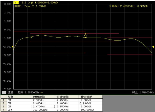
图 3.58 纹波测试结果
