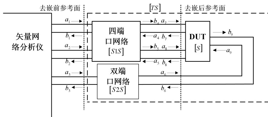
附图 4.10 被测件去嵌入示意图
