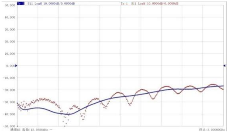
附图 4.8 S11_A (蓝色) 与 S11 (红色) 对比
