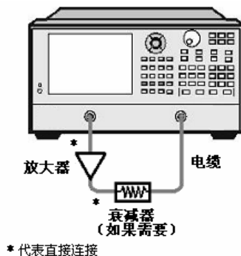
图 8.23 小信号增益和平坦度测量连接
