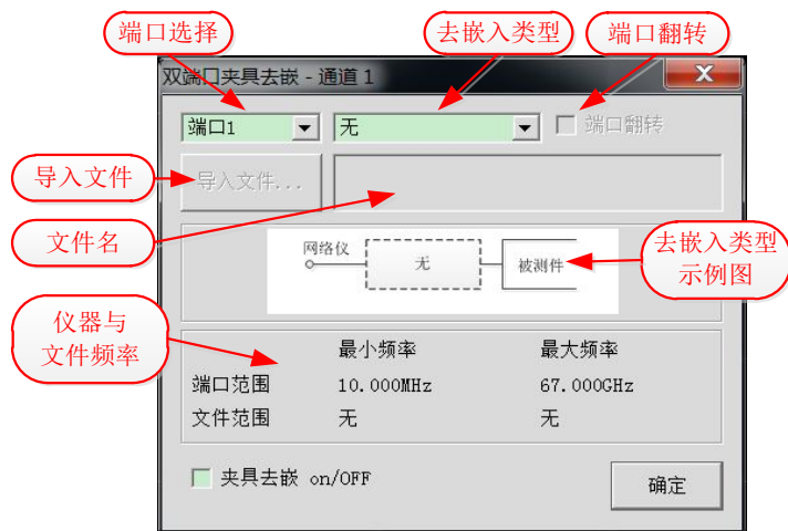
图7.44 双端口夹具去嵌入界面
