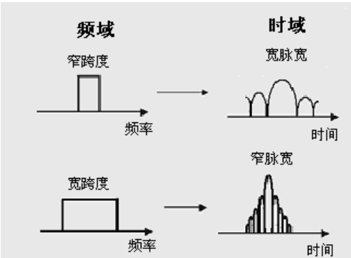
附图 2.3 频域跨度对响应分辨率的影响
