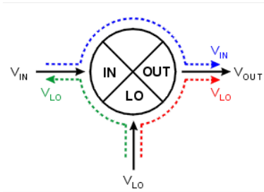
附图 3.7 混频器件信号泄露表示
