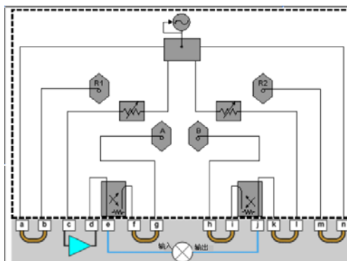
附图 6.31 连接前级放大器示意图
