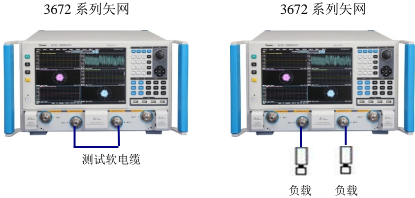
图 11.9 系统动态范围校准测试框图三 图 11.10 系统动态范围校准测试框图四
