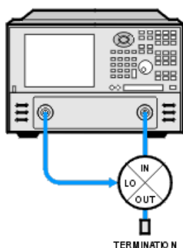
附图 3.8 本振到射频隔离测试
