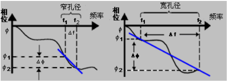
图 8.14 群时延孔径对测量结果的影响
