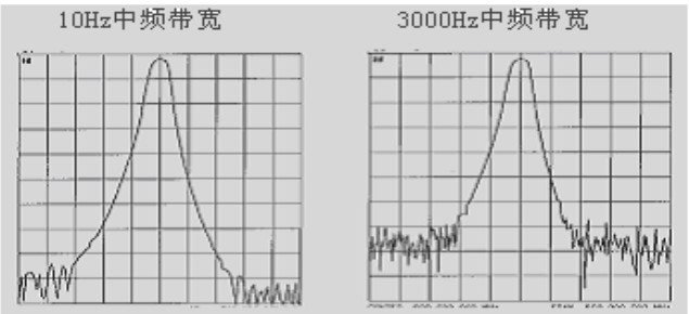
图 6.16 中频带宽对测量结果的影响
