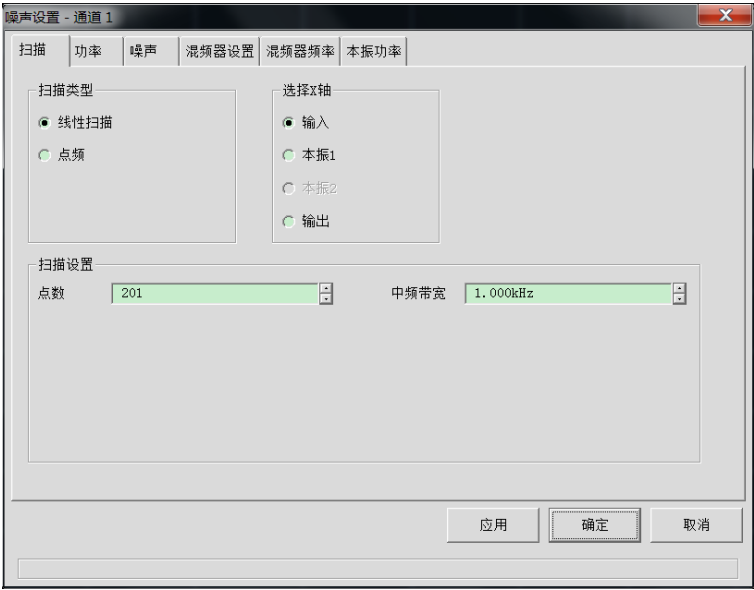
附图 8.22 变频器噪声系数测量频率选项卡
