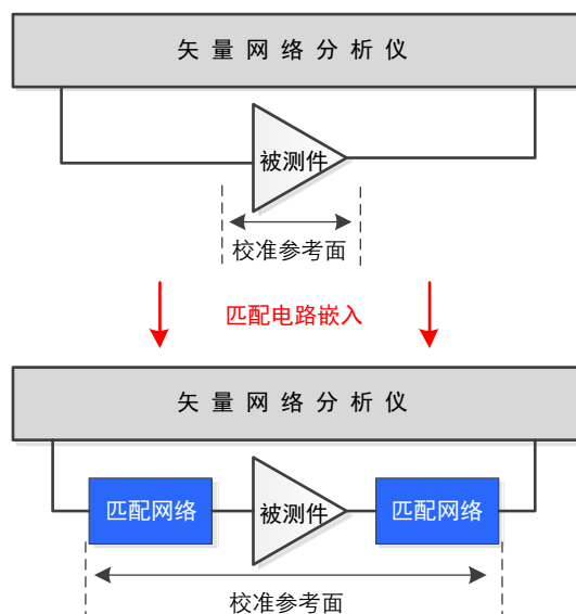
图7.39 匹配电路嵌入示意图
