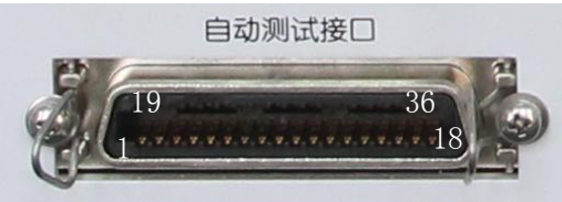
图3.38 自动测试接口连接器
