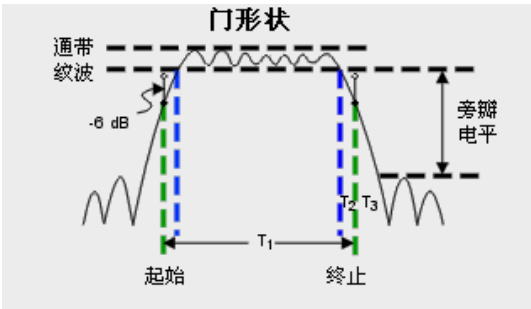
附图 2.13 门形状示意图
