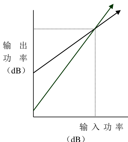
附图 7.2 交截点参数示意图
