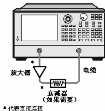
图 8.17 绝对输出功率测量连接
