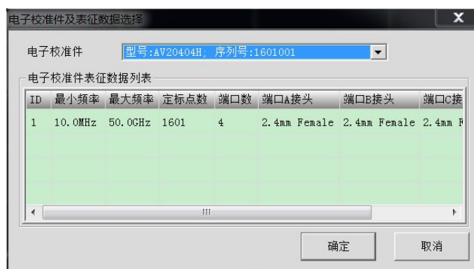
图7.21 校准件及表征数据选择
