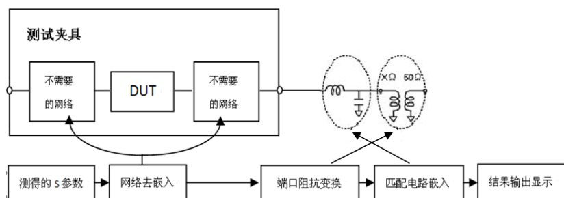
图7.36 夹具仿真器处理流程
