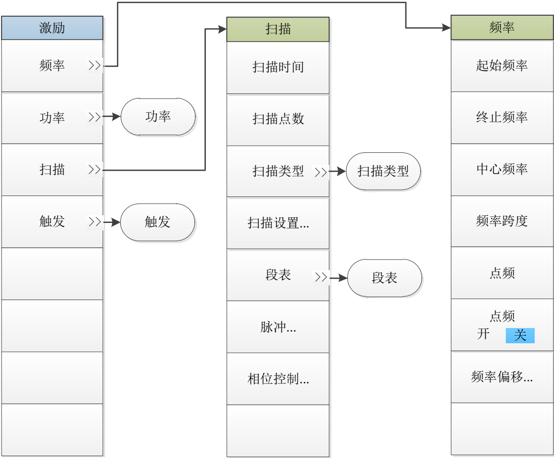
图 5.4 激励菜单一
