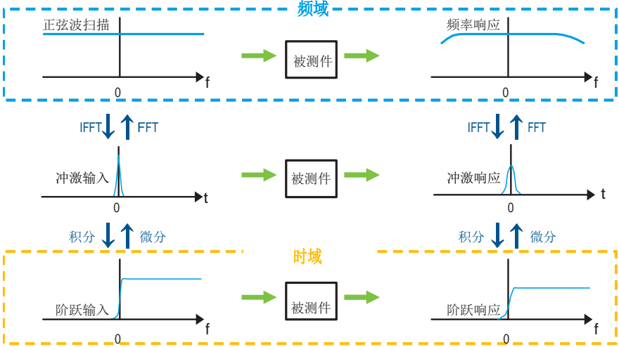
附图 2.27 两类时域反射阻抗测试原理对比
