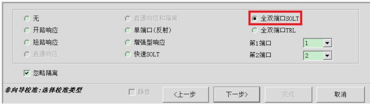
图7.11 为机械校准选择校准类型
