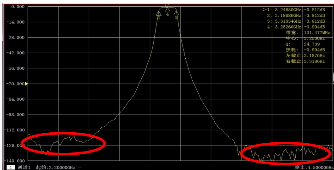
图 2.5 滤波器测量结果
