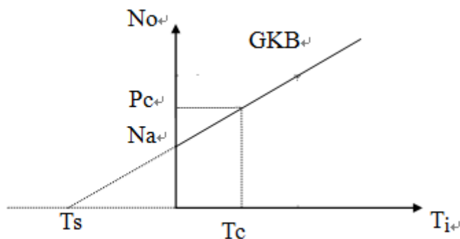
图 8.2 噪声功率对源温度的关系曲线
