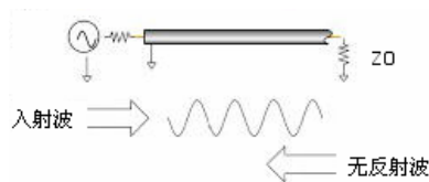
图 8.2 用负载端接的传输线的信号传输
