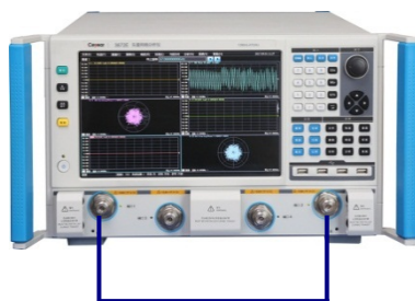
测试软电缆
