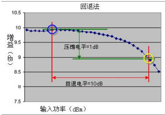
附图5.3 从回退点压缩法计算示意图
