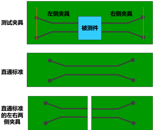
图7.49 差分夹具示意图
