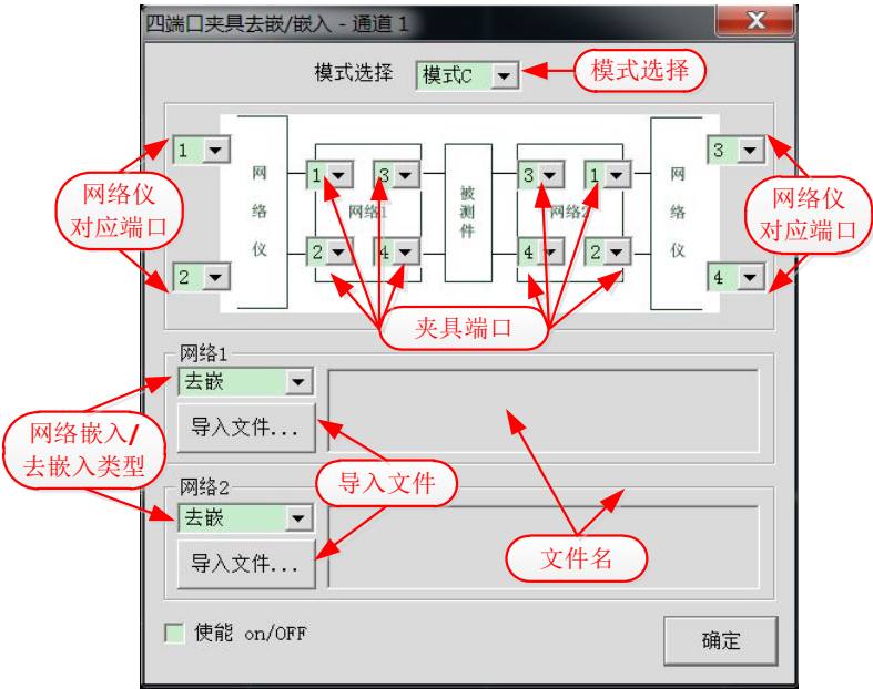
图7.46 四端口夹具嵌入/去嵌入界面
