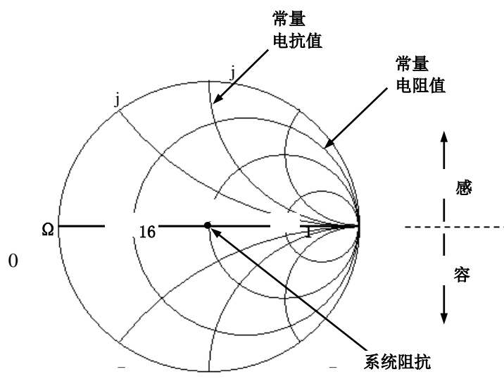
图 4.29 史密斯圆图格式
