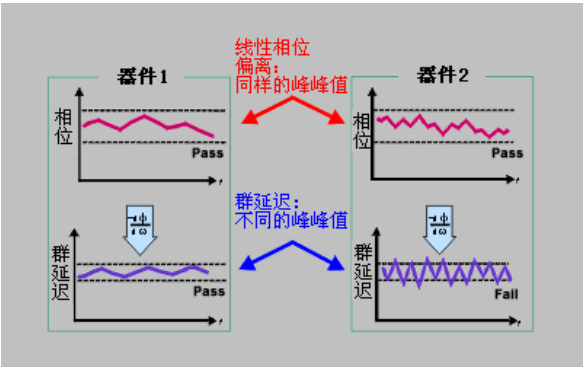
图8.13 群时延与线性相位偏离比较
