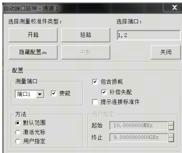
附图9.11 自动端口延伸
