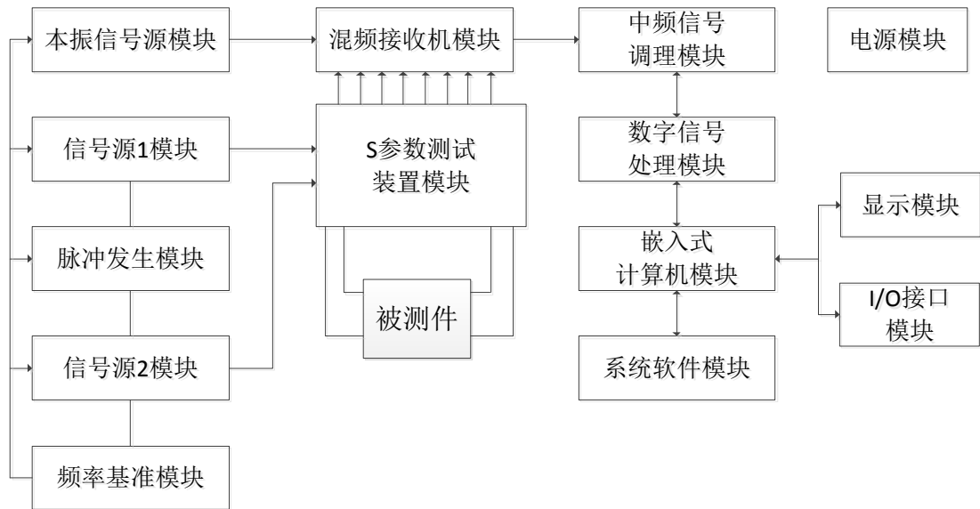
图 10.2 整机原理框图
