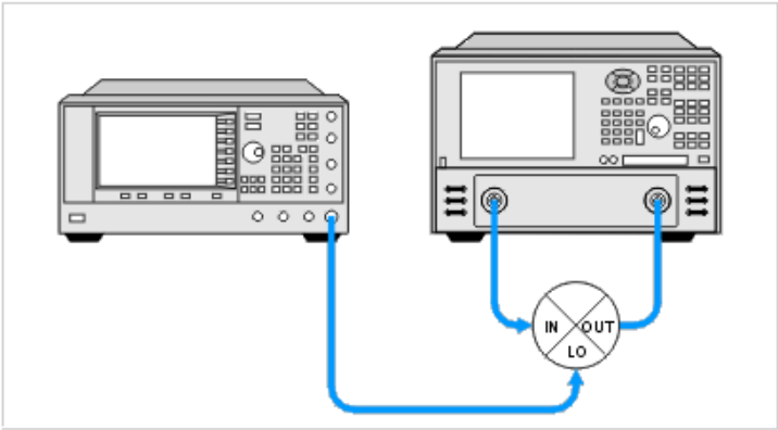
附图 3.6 变频损耗测量连接装置示意图
