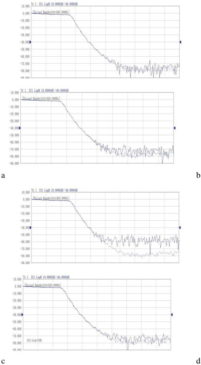
附图 4.11 占空比对动态范围的影响
