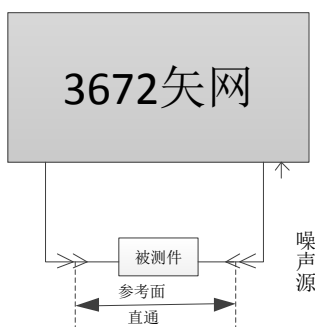
附图 8.16 噪声适配器去嵌
