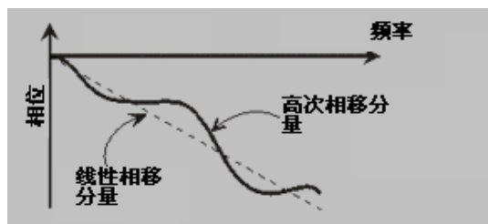
图 8.11 相移与群时延
