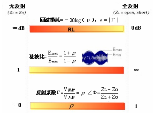
图8.6 各种反射表达之间的关系
