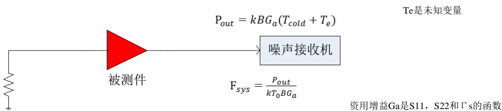
附图 8.5 噪声接收功率公式
