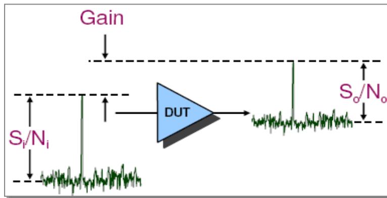
图8.1 噪声系数定义
