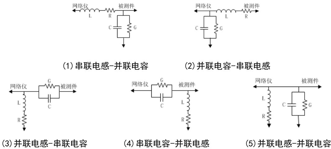
图7.42 嵌入匹配电路的 5 种电路参数模型
