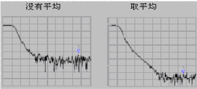
图 6.12 扫描平均对测量结果的影响
