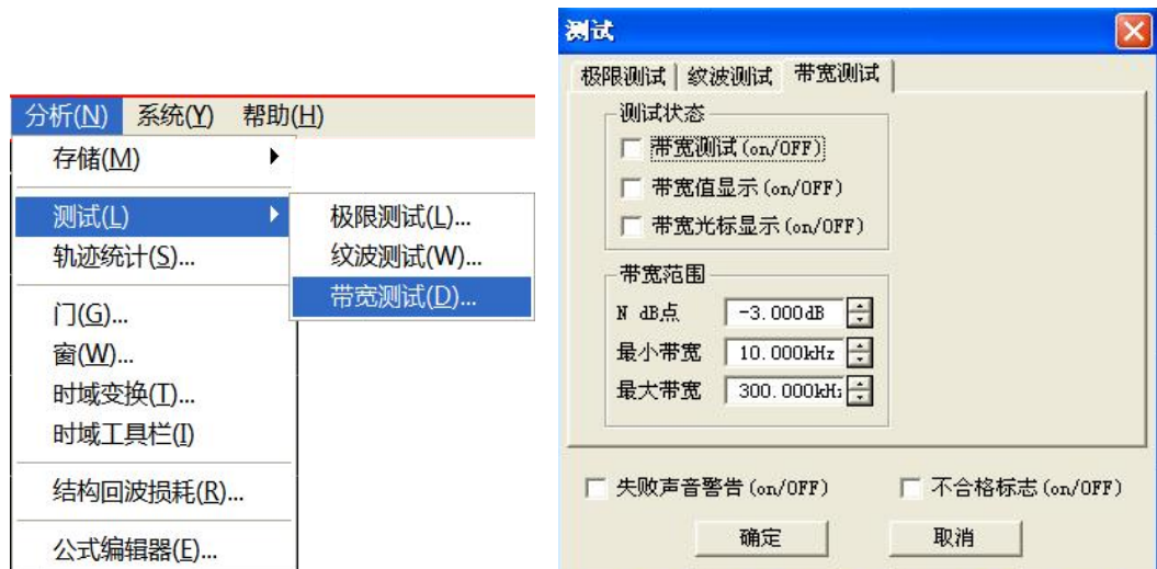
图 3.65 带宽测试对话框
