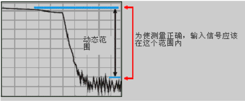
图 6.3 动态范围
