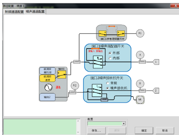
附图8.24 噪声通道配置
