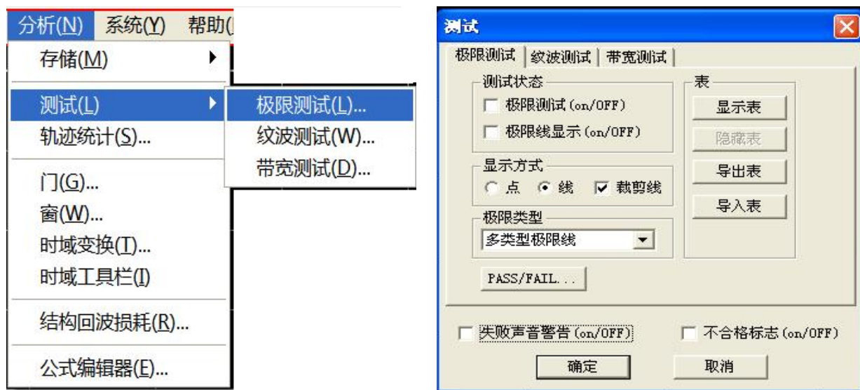
图 3.60 极限测试
