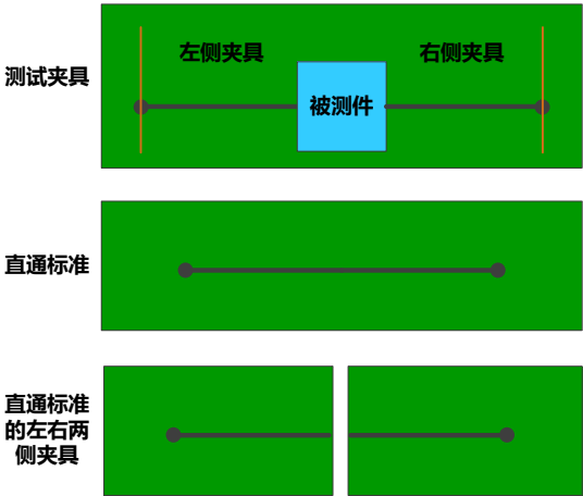
图7.48 单端夹具示意图
