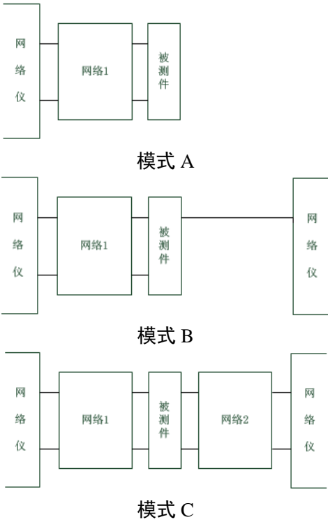
图7.47 夹具嵌入/去嵌入的 3 种模式
