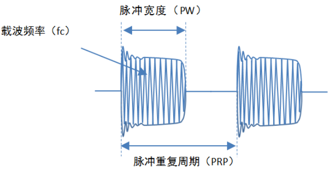
附图 4.1 脉冲信号时域波形
