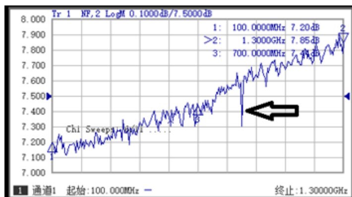
附图 8.18 噪声系数测量可能受到空间干扰
