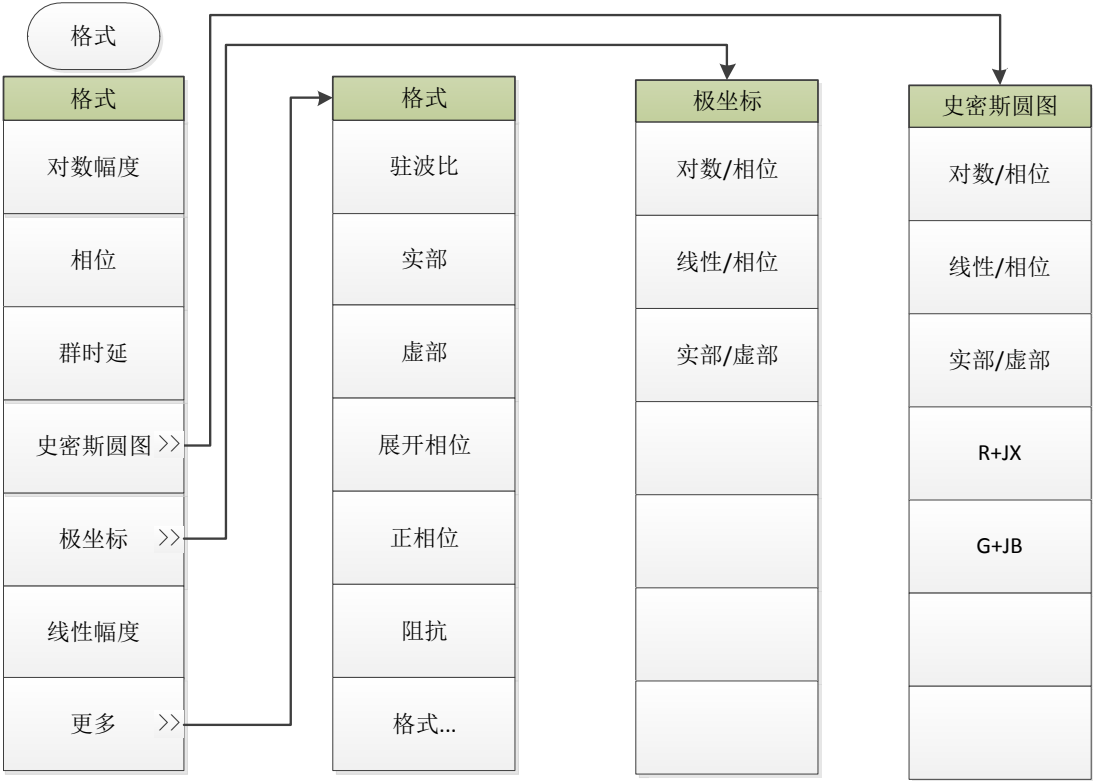
图 5.9 响应菜单三
