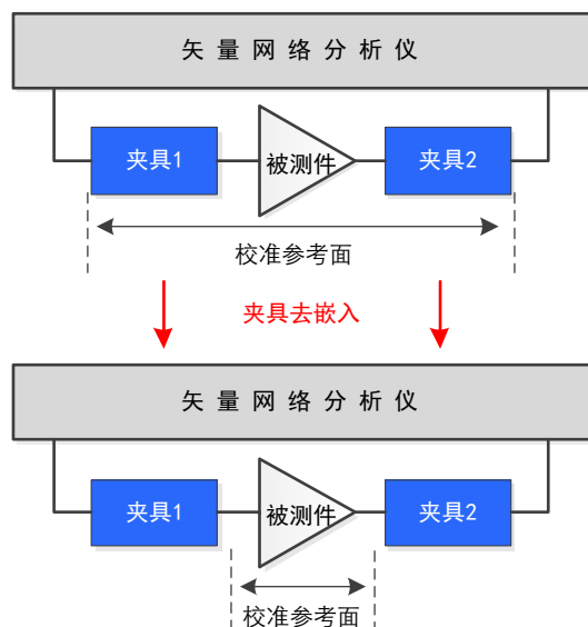
图7.43 夹具去嵌入示例图
