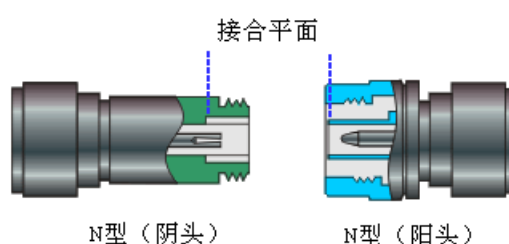
图 3.8 校准平面
