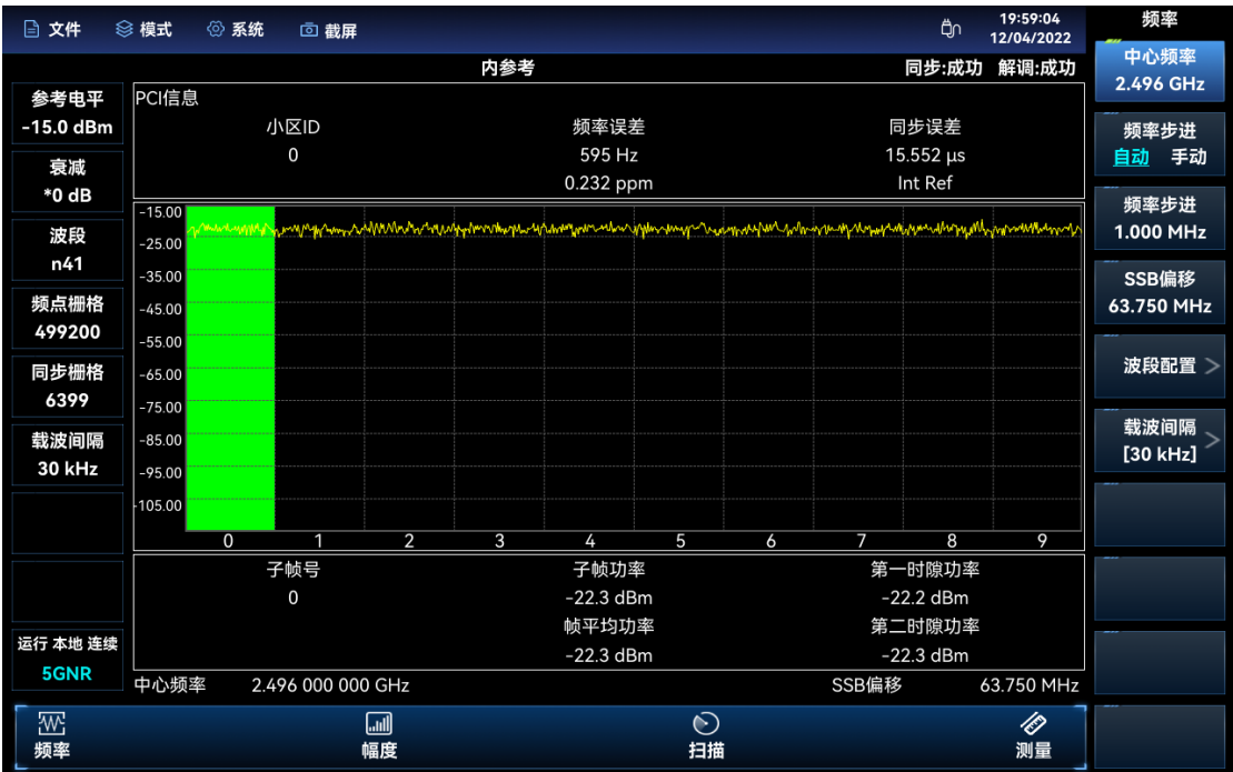
图 17.8 功率 VS 时间显示界面
