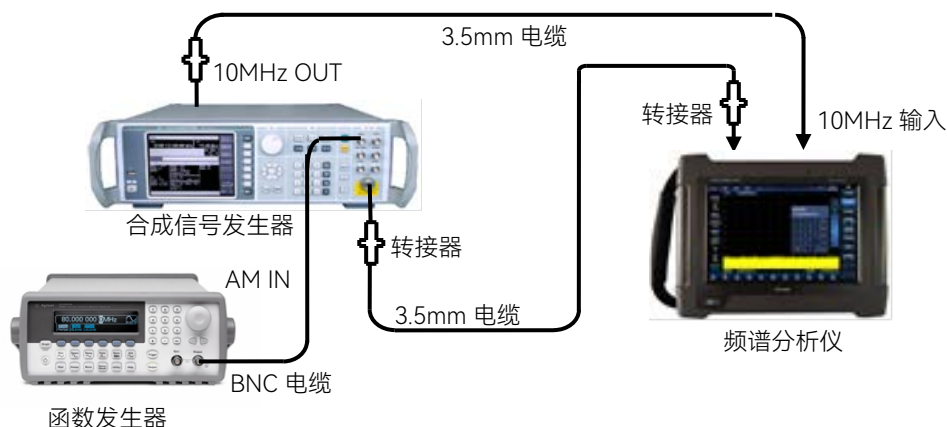
图 19.5 扫描时间准确度测试设置
