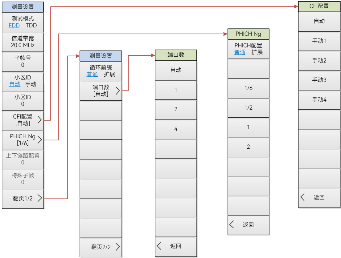
图 16.14 LTE 分析模式触发菜单结构框图
