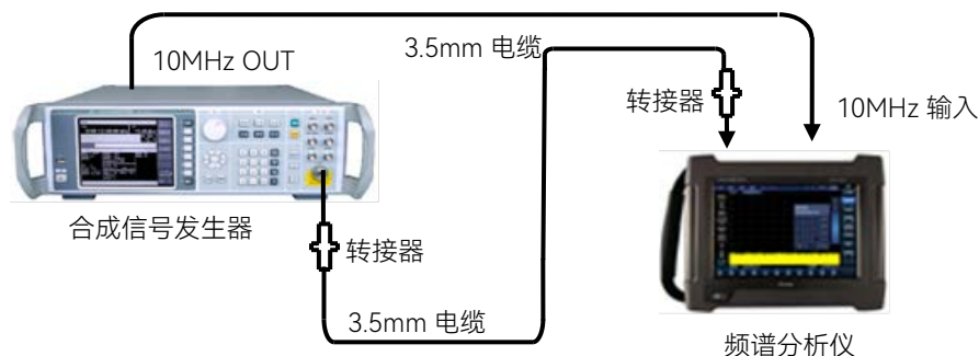
图 19.4 扫频宽度准确度测试设置
