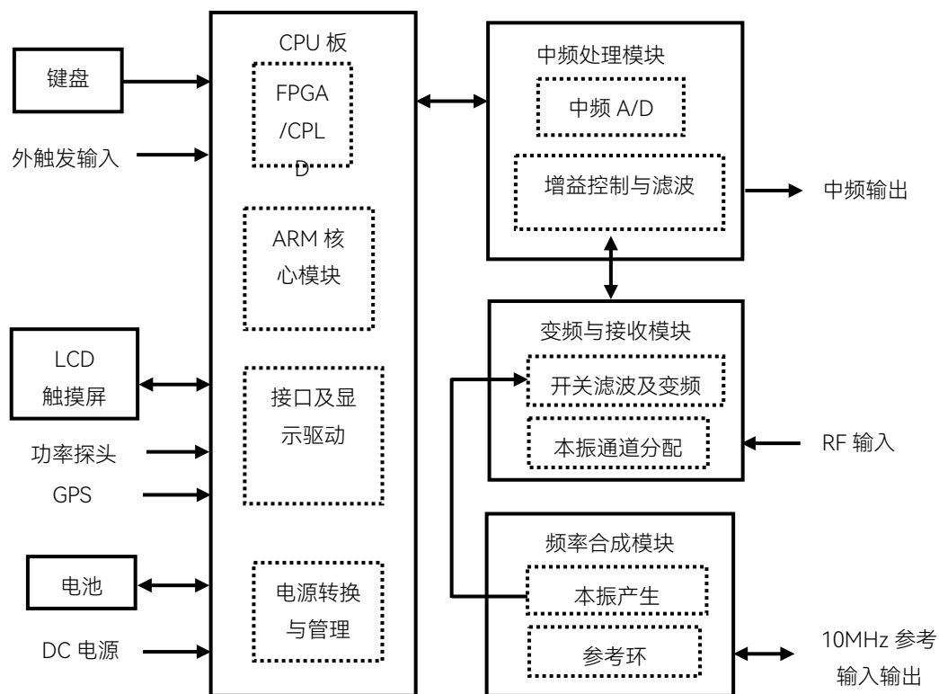
图 18.1 整机硬件总体方案框图
