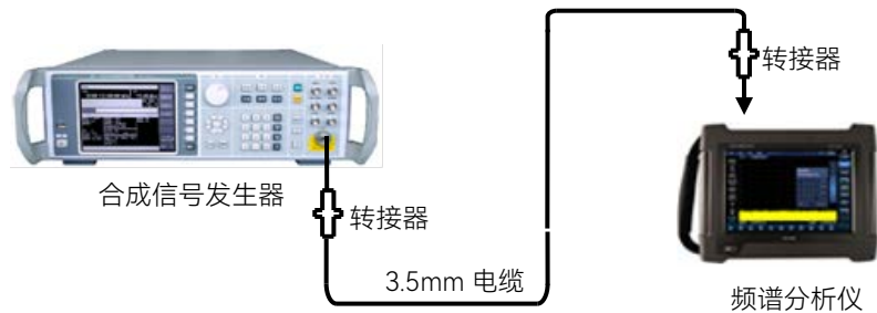
图 19.3 频率读出准确度测试框图
