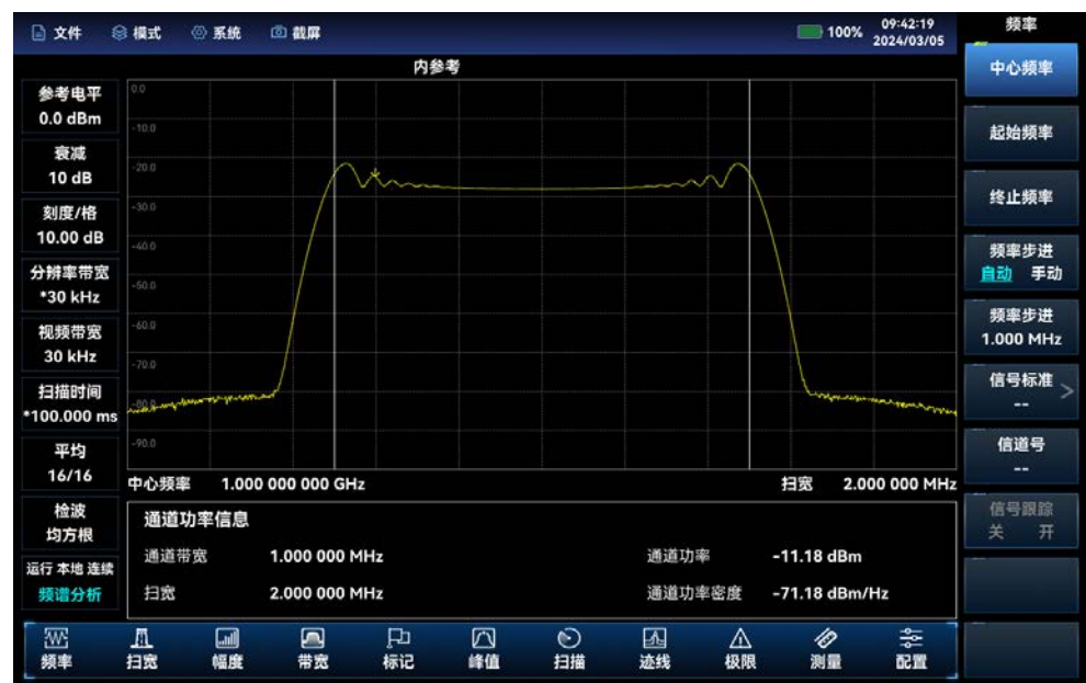
图 4.2 调频信号通道功率测量
