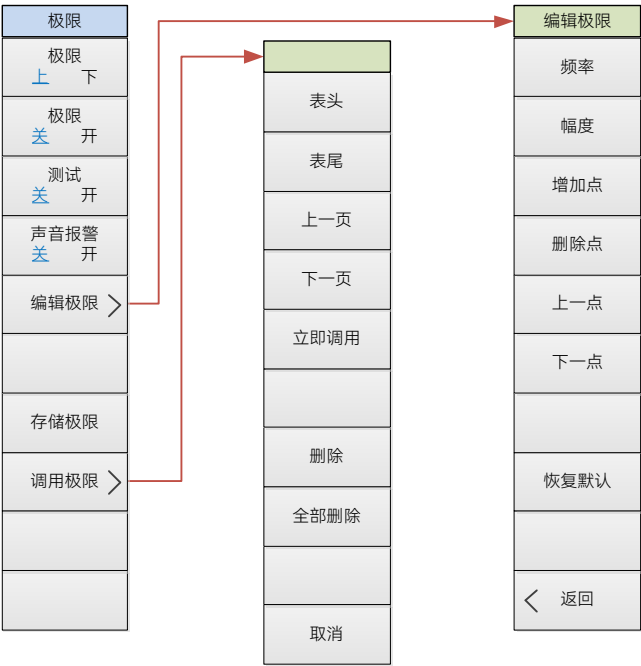
图 11.13 实时频谱模式极限菜单结构框图
