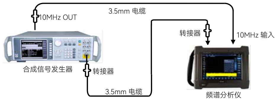
图 19.8 边带噪声测试示意图
