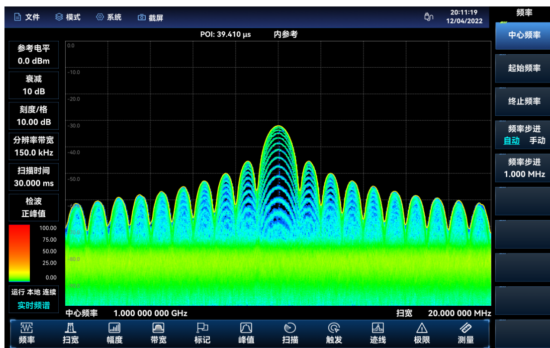
图 11.1 余辉图示意图
