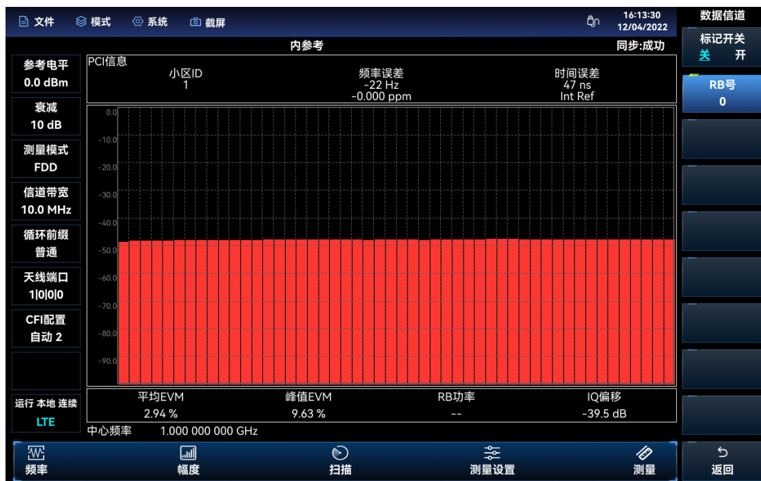
图 16.2 数据信道测试结果
