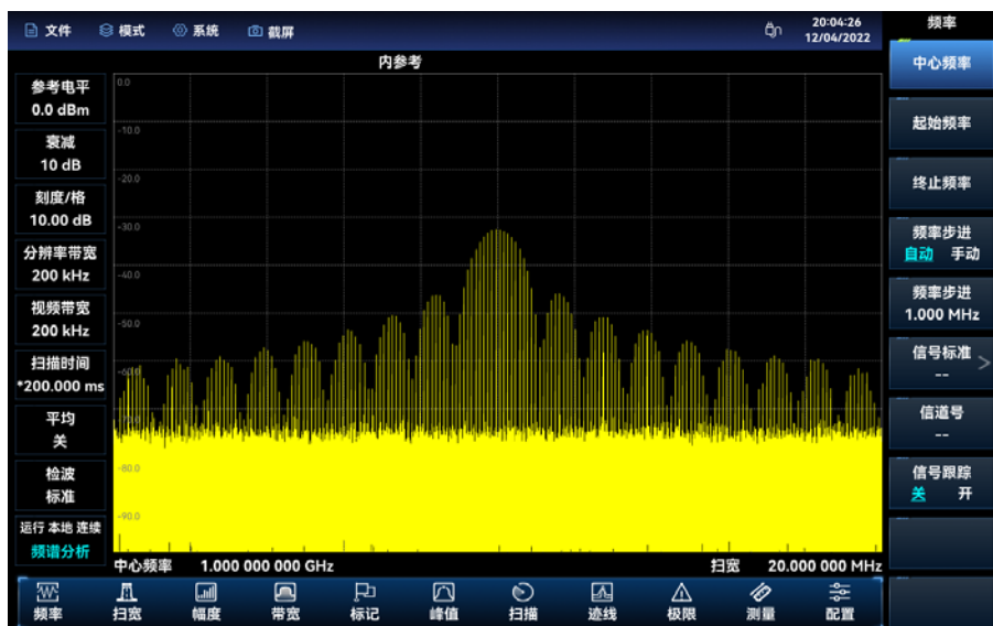
图 4.20 主瓣和旁瓣
