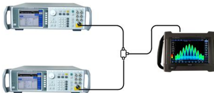
图 3.25 测试两个输入信号的仪器连接图
