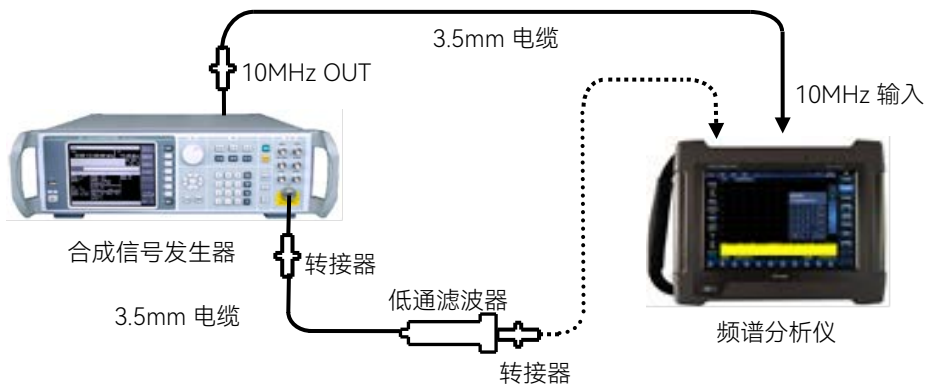
图 19.10 二次谐波失真测试设置
