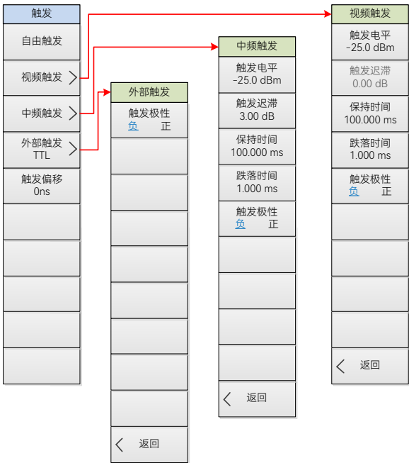
图 14.9 IQ 分析模式触发菜单结构框
