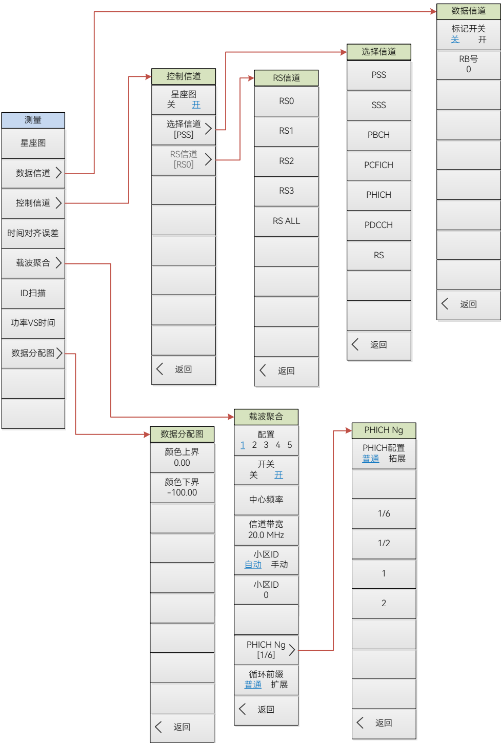
图 16.15 LTE 分析模式测量菜单结构框图
