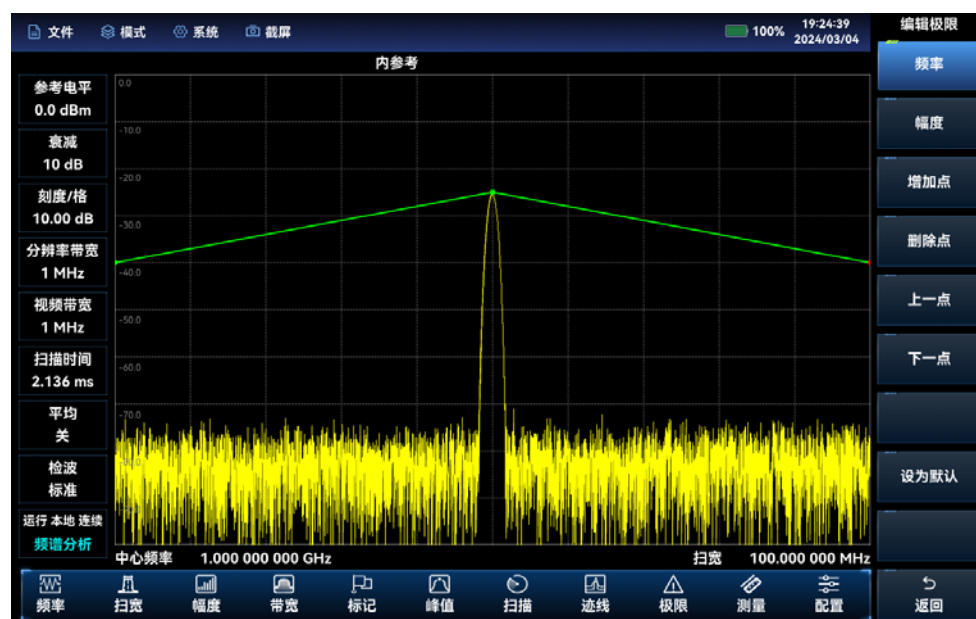
图 4.28 频谱发射模板测量
