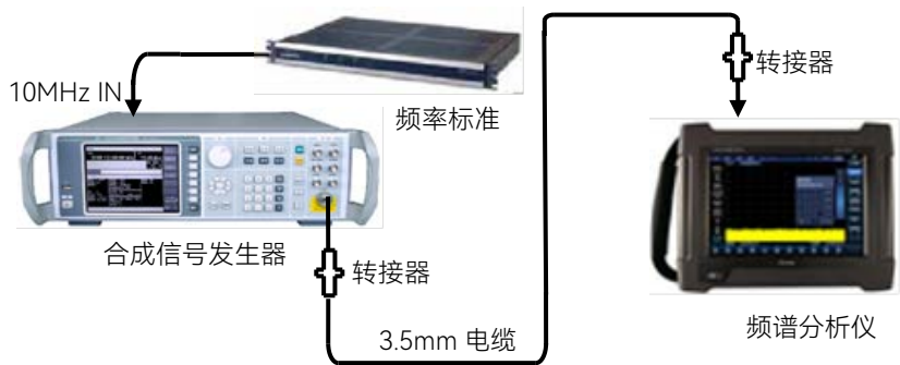
图 19.1 频率参考准确度测试
