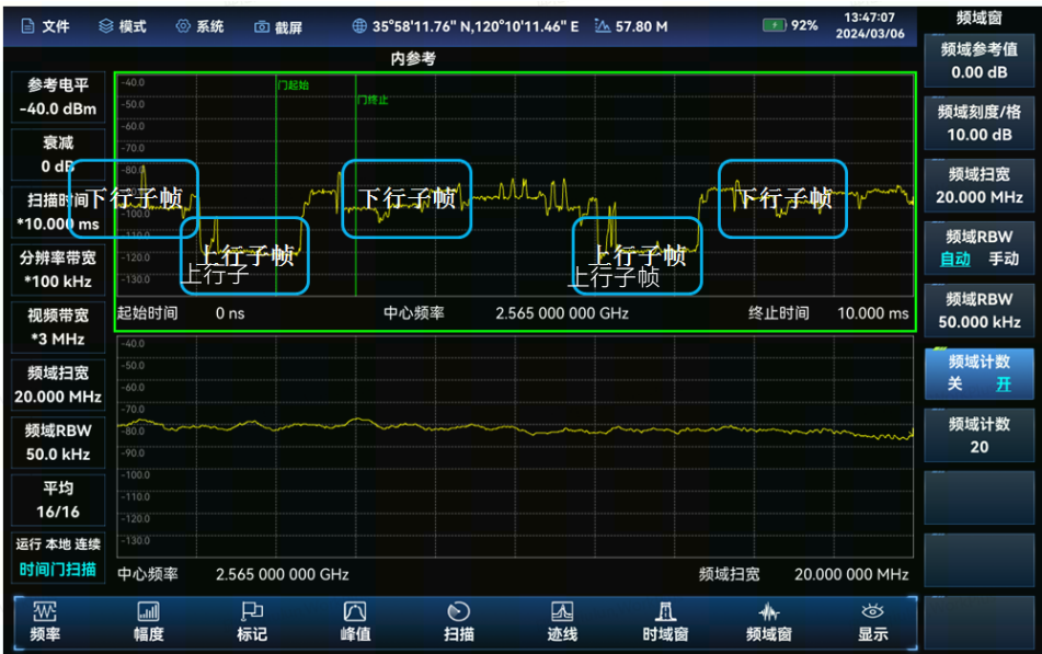
图 13.1 TDD 信号干扰排查示意图
