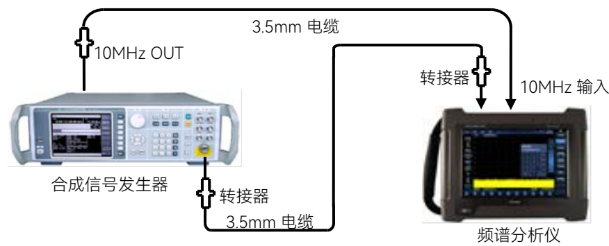
图 19.13 镜像、多重和带外响应测试设置
