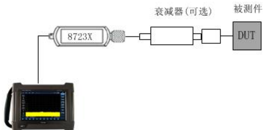
图 8.1 功率测量结构图
