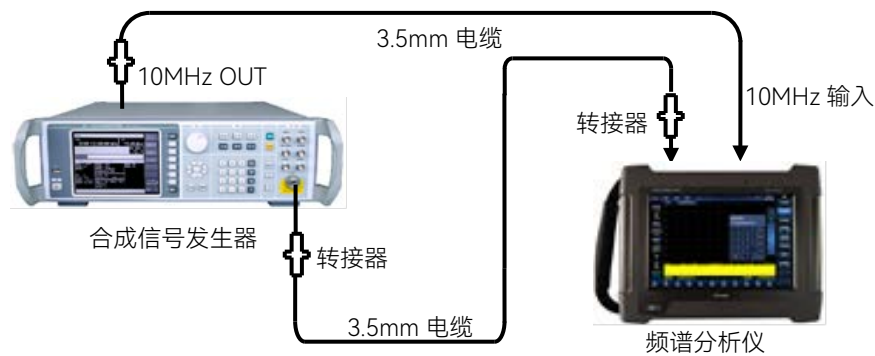
图 19.6 分辨率带宽测试设置
