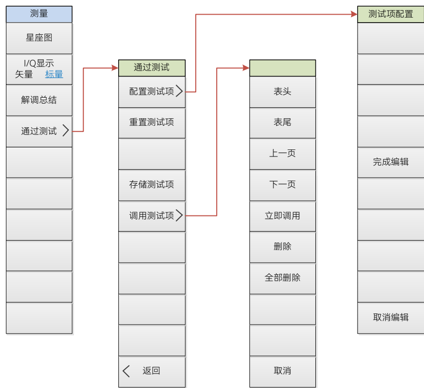
图 15.7 GSM/EDGE 模式测量菜单结构框图
