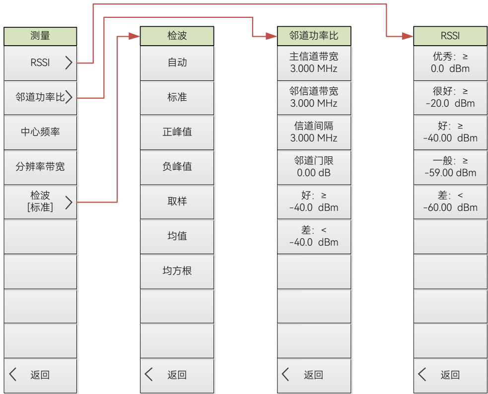
图 4.42 频谱分析模式测量菜单结构框图（续 2）
