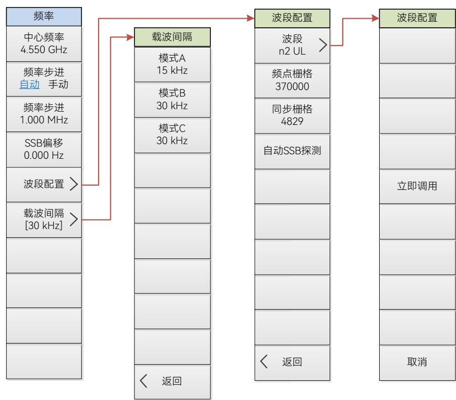
图 17.12 5GNR 模式频率菜单结构框图
