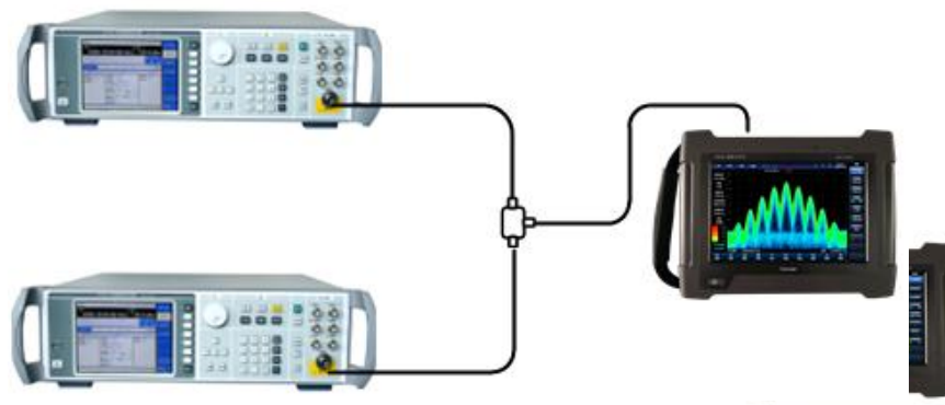
图 4.5 连接三阶交调失真测量系统
