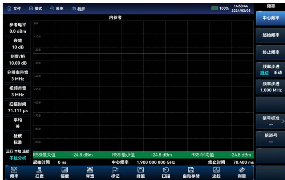
图 5.2 干扰分析 RSSI 测试图
