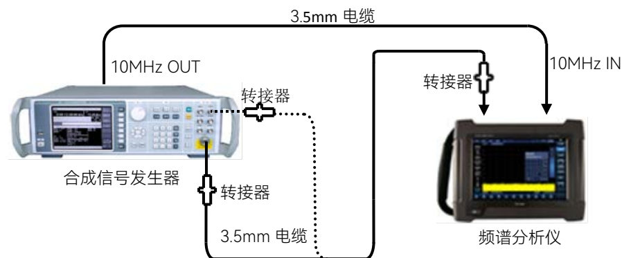
图 19.2 频率范围的测试
