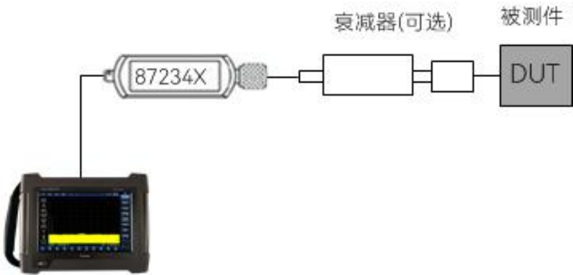
图 12.1 功率测量结构图
