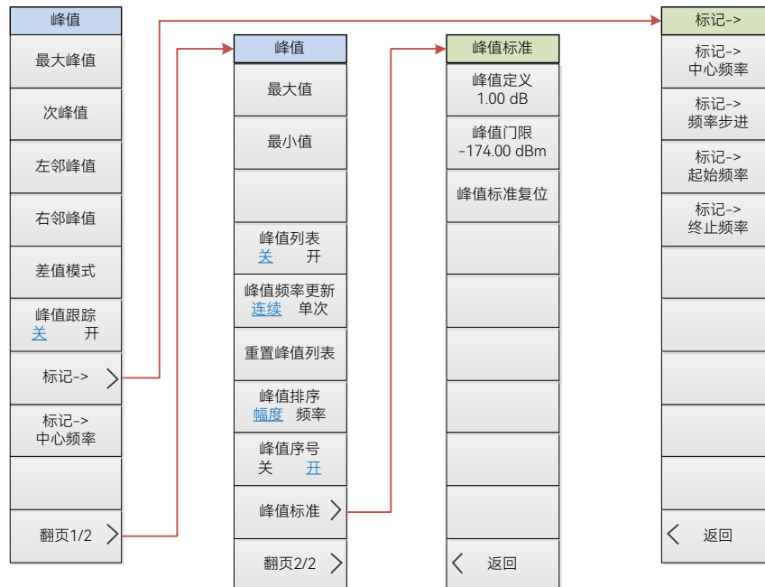
图 4.36 频谱分析模式峰值菜单结构框图
