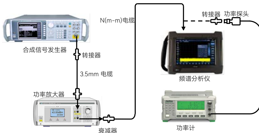
图 19.19 最大安全输入电平测量
