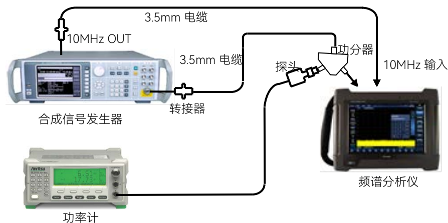
图19.15 参考电平不确定度与刻度保真度测试设置
