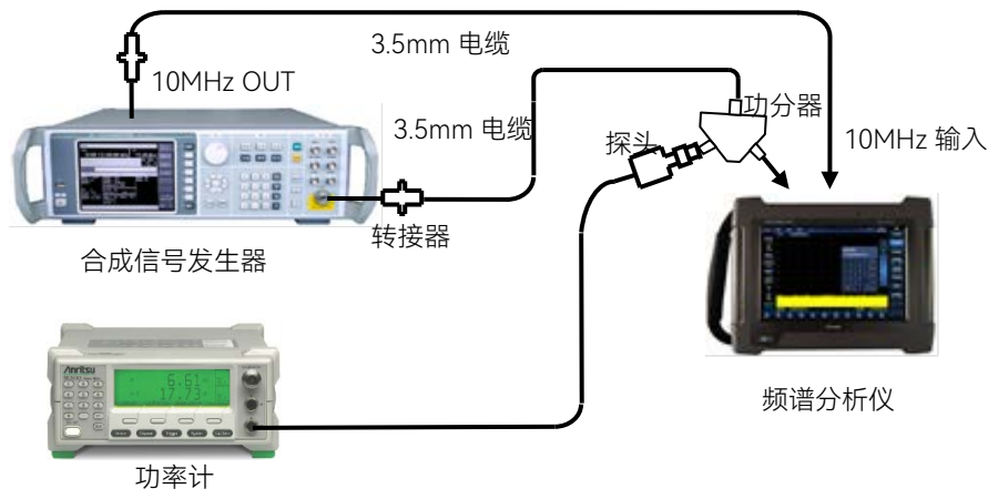
图 19.16 总电平不确定度测试设置
