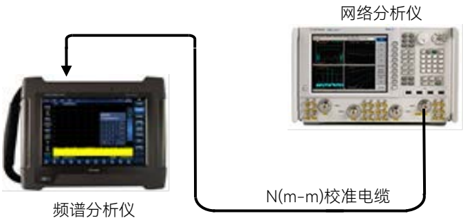
图 19.18 输入端口电压驻波比测试
