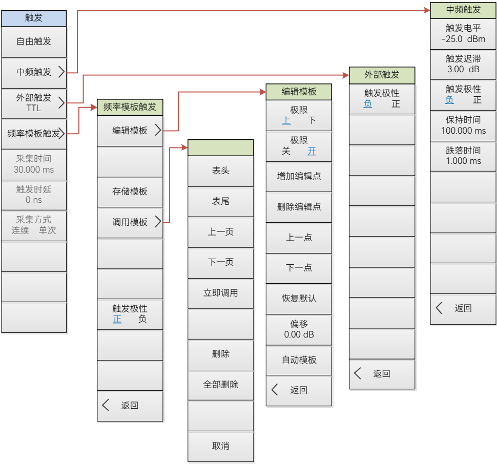
图 11.10 实时频谱模式触发菜单结构框图
