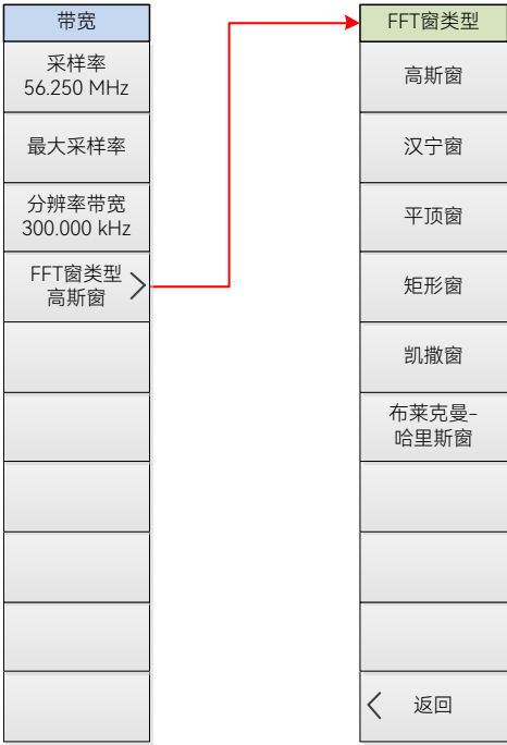
图 14.3 IQ 分析模式带宽菜单结构框图
