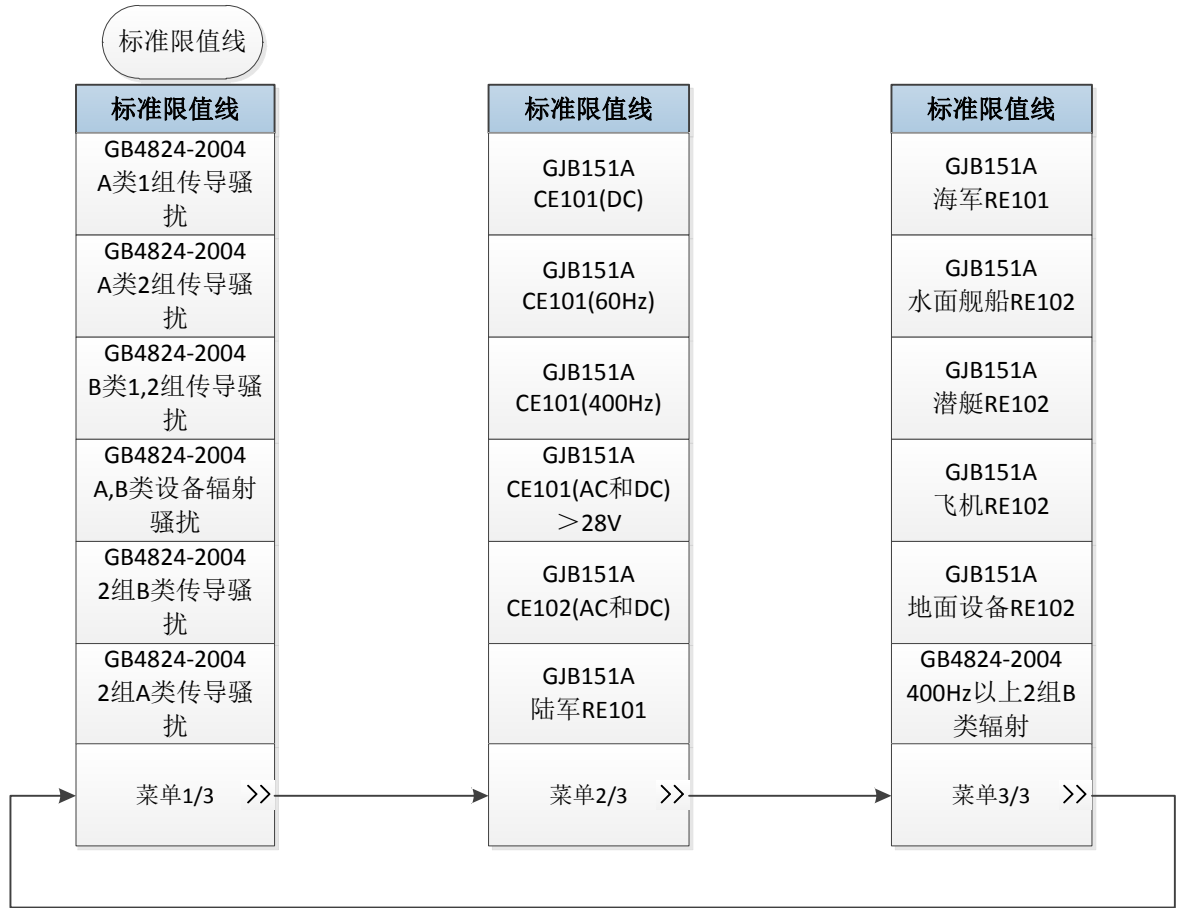
图 3-11 测量设置菜单
