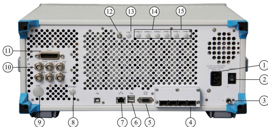
图 3.14 3915 后面板
