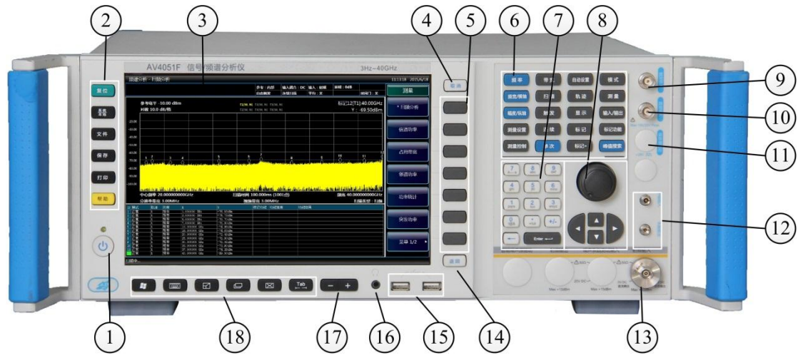
图 3.12 3915 前面板
